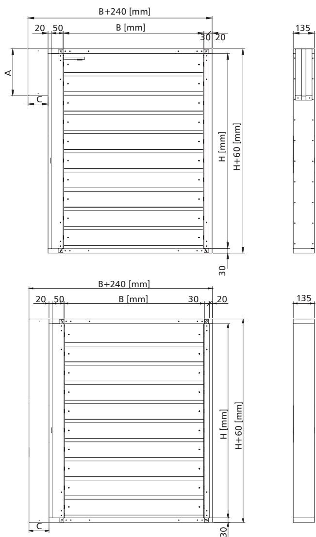
LC - długa obudowa siłownika
